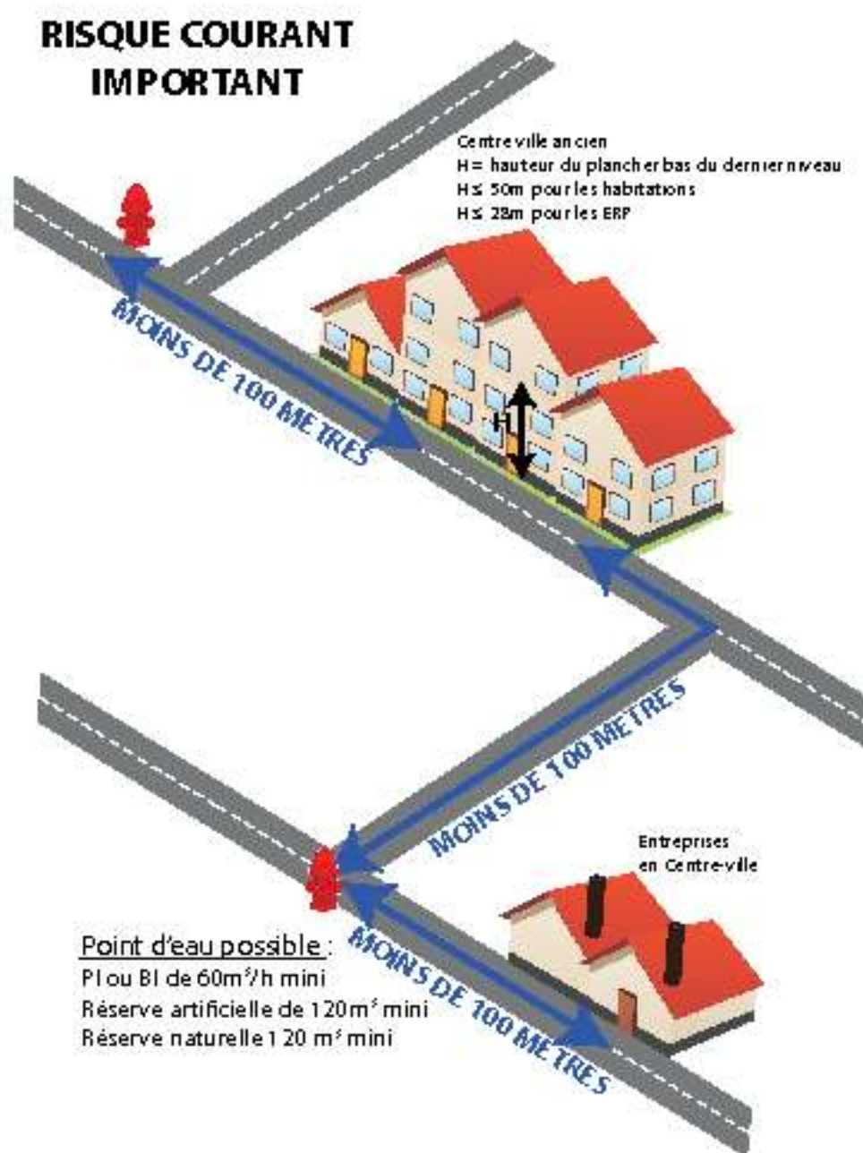
Figure 5 : schéma de principe pour la couverture du risque courant important
