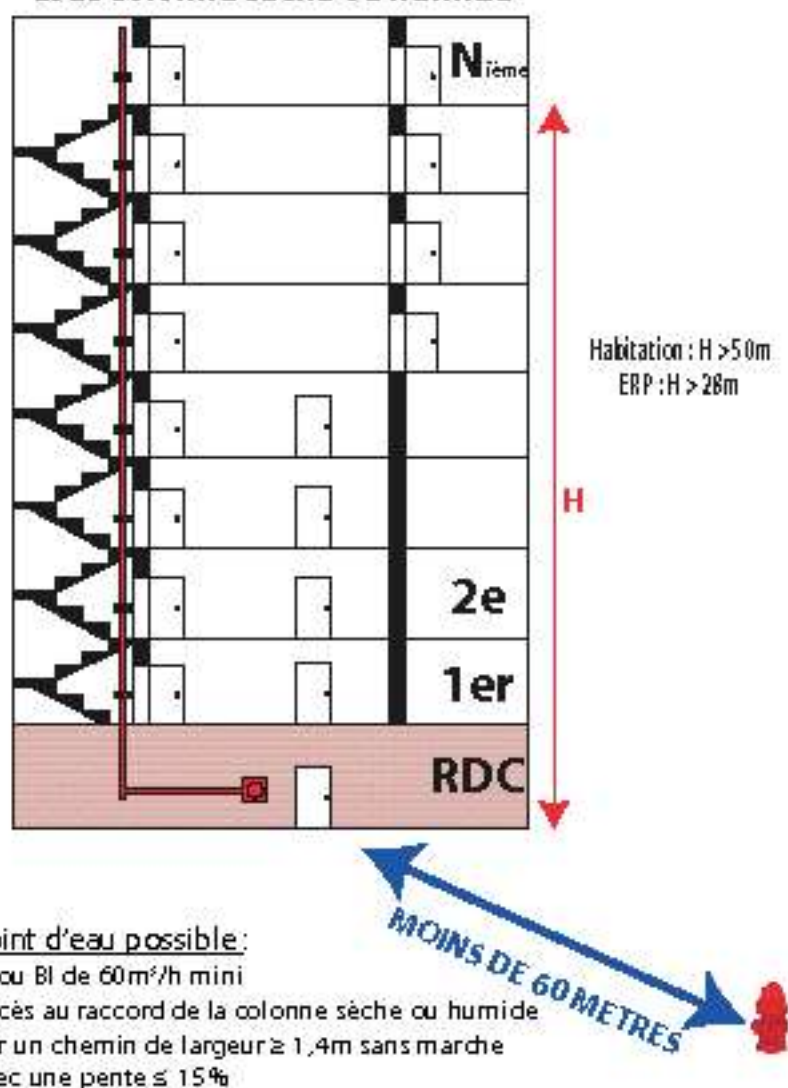
Figure 8 : Schéma de principe pour la couverture d'un IGH avec colonne sèche ou humide imposée
