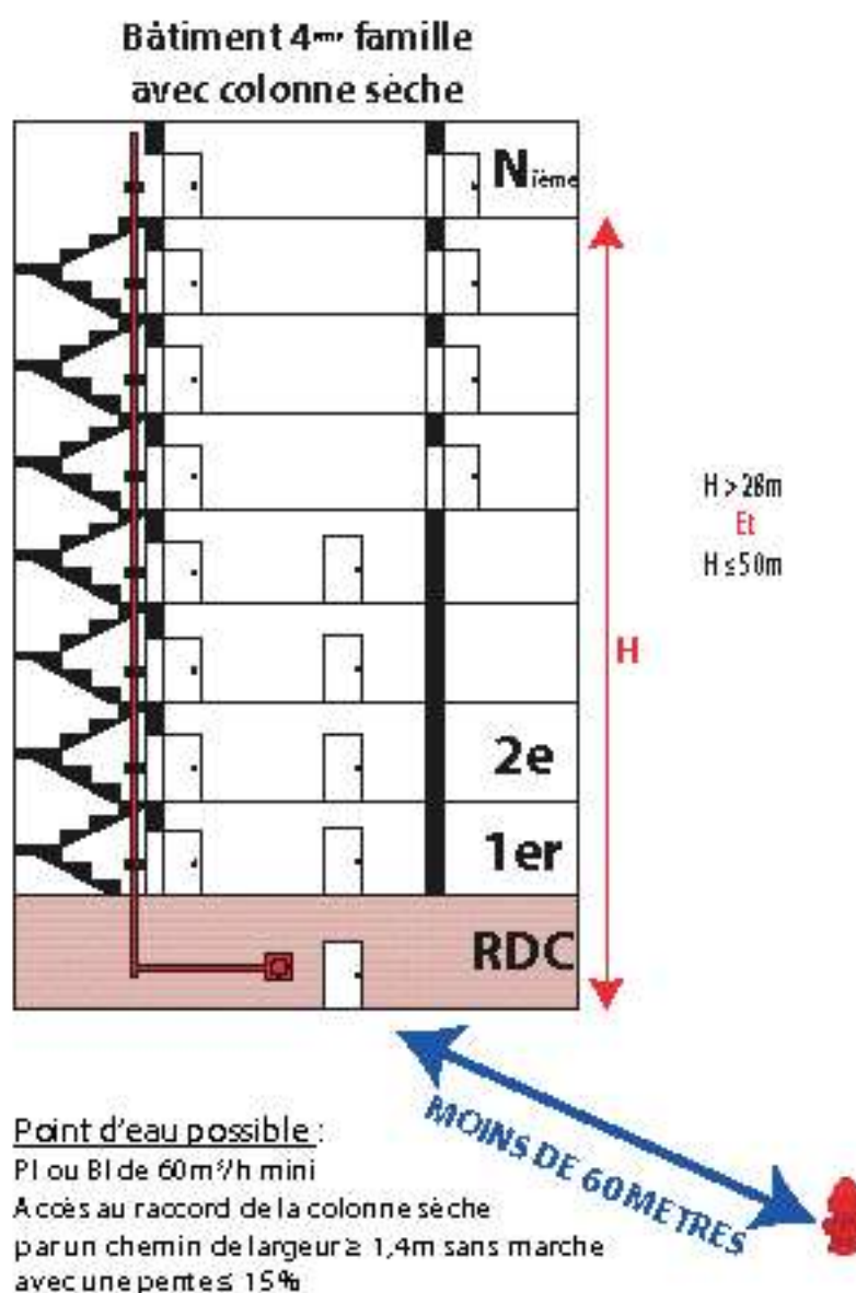
Figure 7 : Schéma de principe pour la couverture d'une habitation 4 ème famille avec colonne sèche imposée
